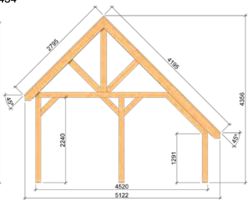
Zijaanzicht: Kapschuur XXL
